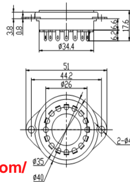
管座图 (CE243, 单位mm)
