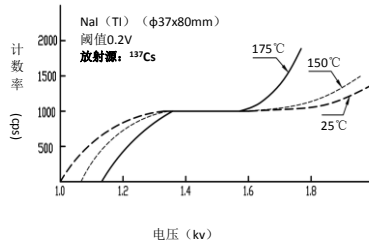
典型坪曲线
