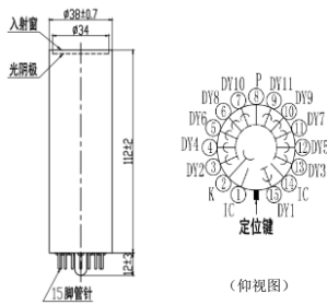
外形图 (单位mm)
